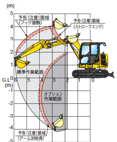
■ 作業範囲図(ロングアーム)
