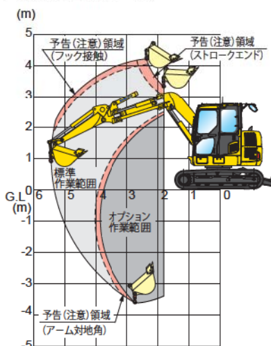
■ 作業範囲図(標準アーム)
